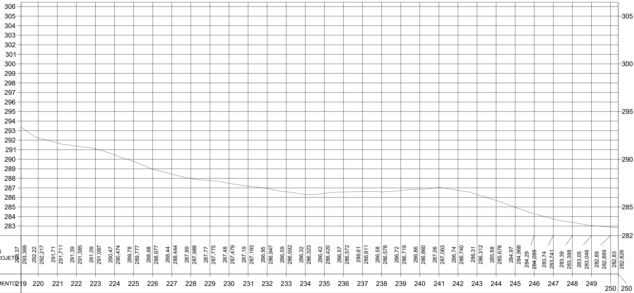
PERFIL TRECHO 1: MORADA NOVA DOS NUNES
