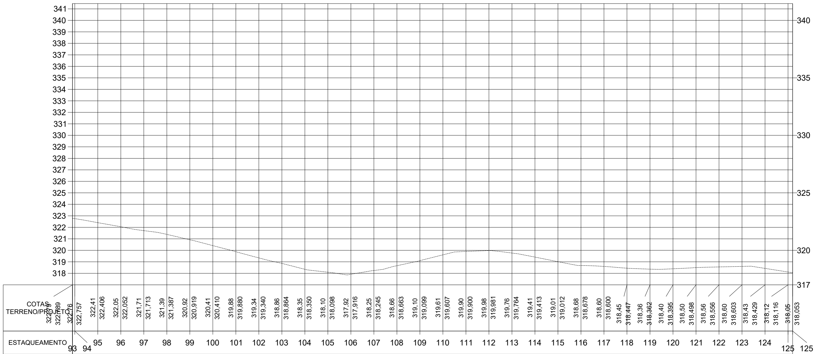
PERFIL TRECHO 1: MORADA NOVA DOS NUNES
