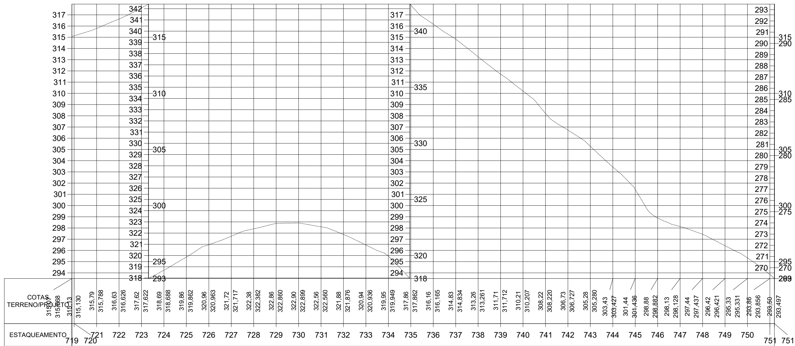
PERFIL TRECHO PEREIRA NOVA DOS NUNES
