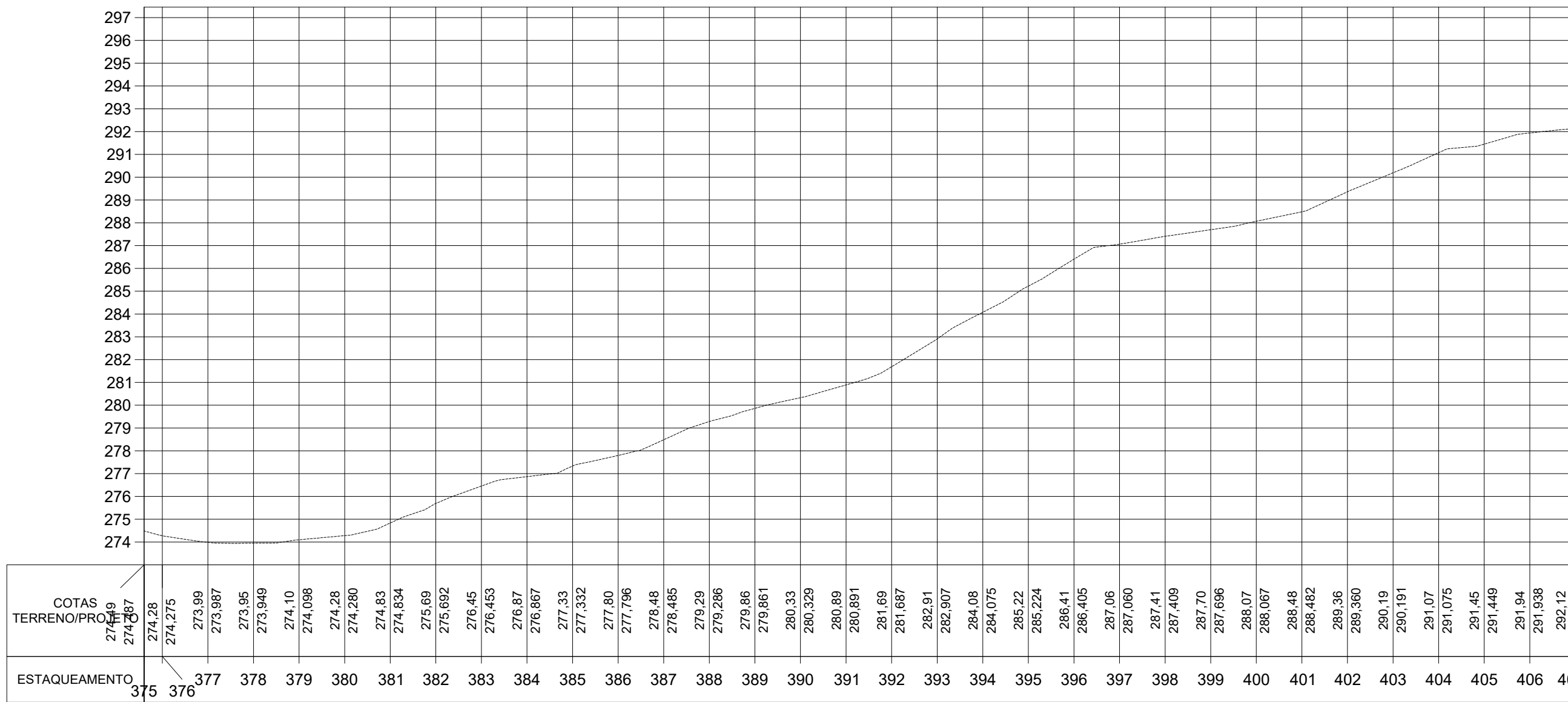
PERFIL TRECHO 1: MORADA NOVA DOS NUNES
