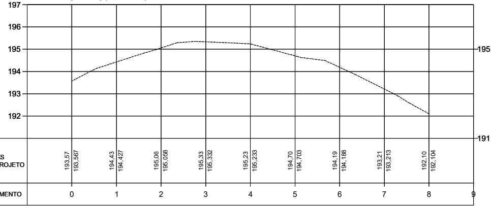
PERFIL RUA PROJETADA 01
