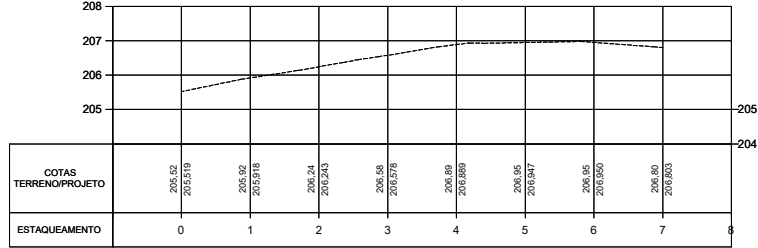
PERFIL RUA CARRO VELHO
